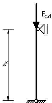
einteilige Stütze
